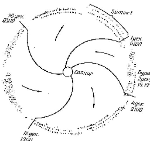
Рис. 8. Четыре сектора магнитного поля Солнца. Пробразы свастики и Креста Христова.
