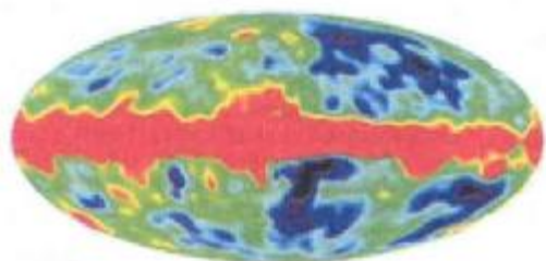
Рис. 6. Распределение материи и энергии в первичной Вселенной. Красный цвет – реликтовое излучение.
