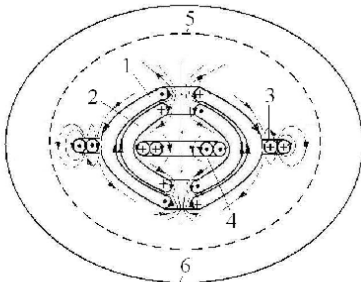
Рис. 2. Модель структуры остова («ядра») Солнца. 1, 2 – сфероидальные правая и левая подоболочки; 3, 4 – внешние и внутренние орбитали, состоящие из пар право-левых вихрей; 5 – условная граница атмосферы оболочки, ее радиус равен радиусу центрального ядра Солнца ( \sim R_{\odot}/4 ); 6 – внешняя граница фотосферы Солнца – радиус R_{\odot} = 7 \cdot 10^{10} см. Пунктирными стрелками показаны направления циркуляций магнитного поля.
