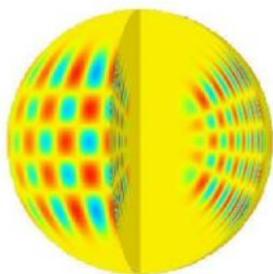
Рис. 5. Симметрия деформационных радиальных колебаний Солнца.
