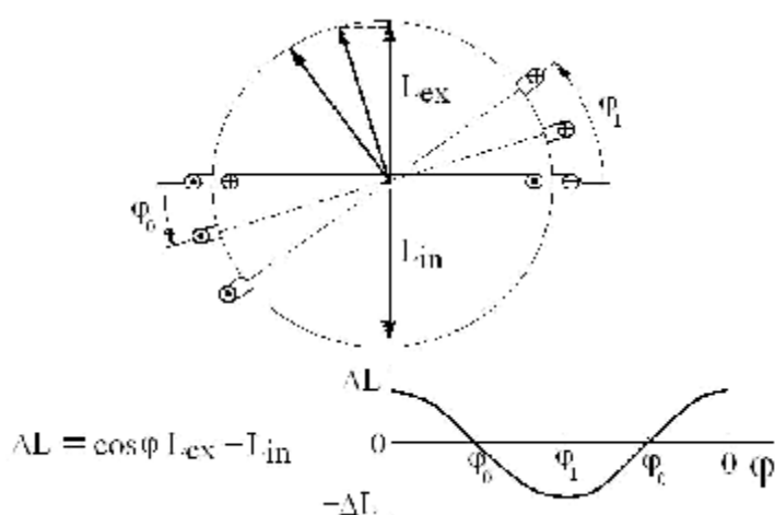
Рис. 3. Схема гармонических колебаний внешней орбитали Солнца (момент импульса L_{ex} ) относительно неподвижной внутренней орбитали ( L_{in} ). Период колебаний – изменения угла от 0 до \varphi_1 составляет \sim 22 года. При значении угла \varphi_0 происходит переполюсовка магнитного поля Солнца. Угол \varphi_0 может быть равен углу наклона оси вращения Солнца к плоскости эклиптики ( 7^{\circ} 15' ).
